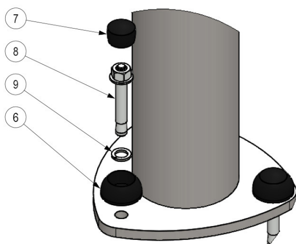
DÉTAIL A
