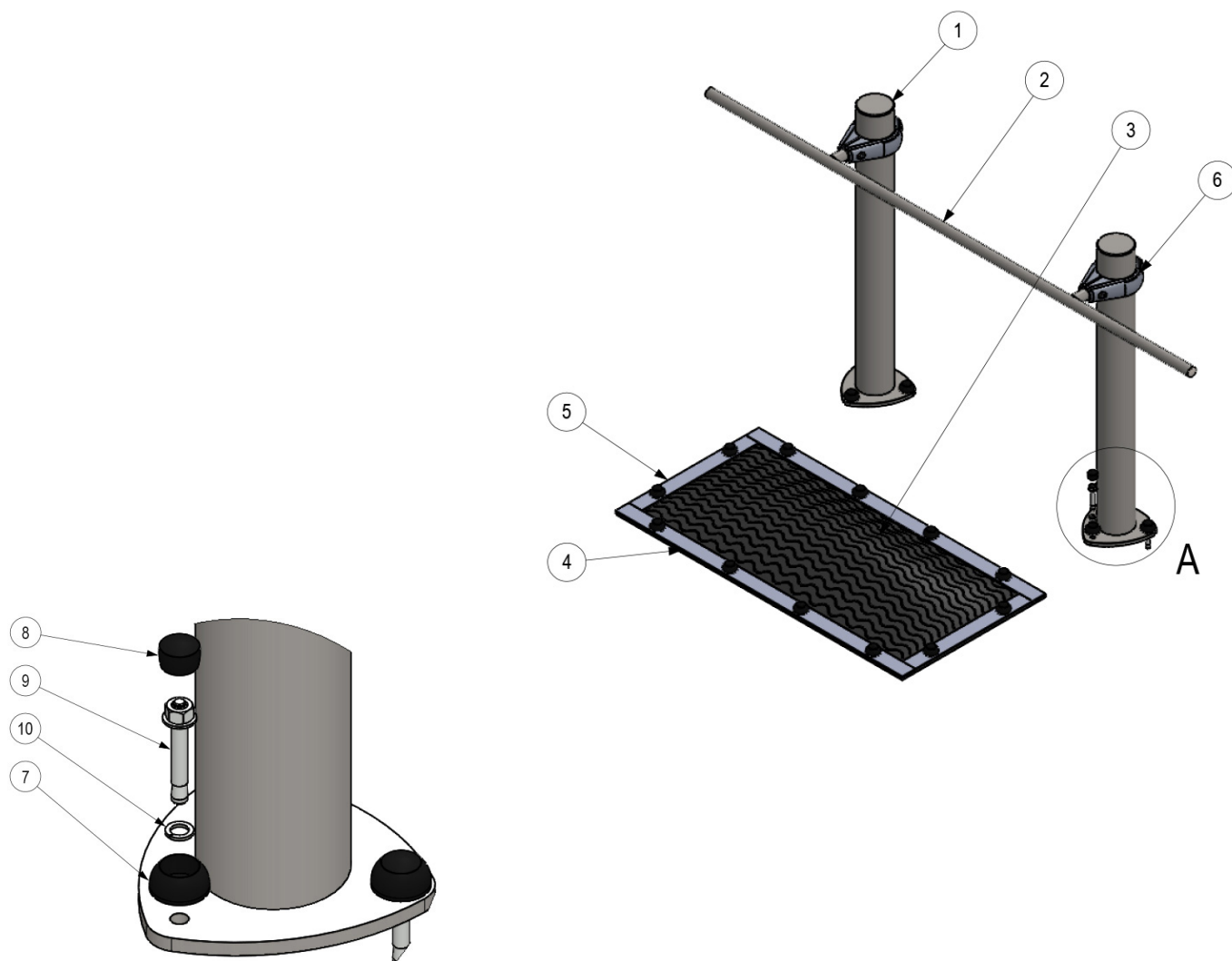
DÉTAIL A
