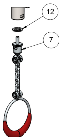
DÉTAIL B
