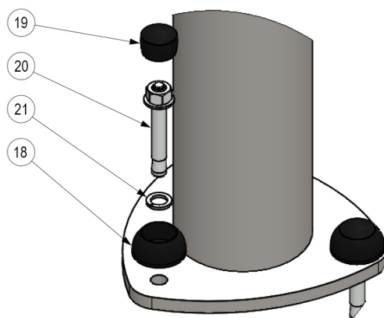
DÉTAIL C
