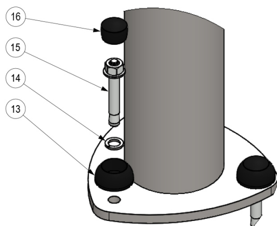
DÉTAIL B
