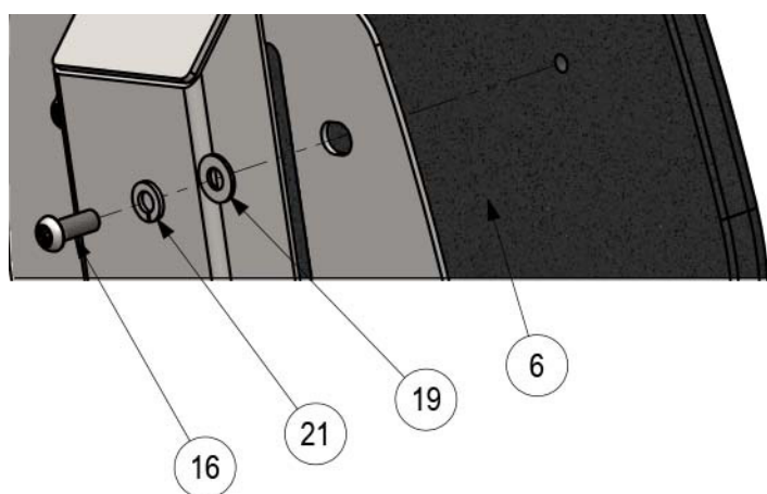
DÉTAIL B
