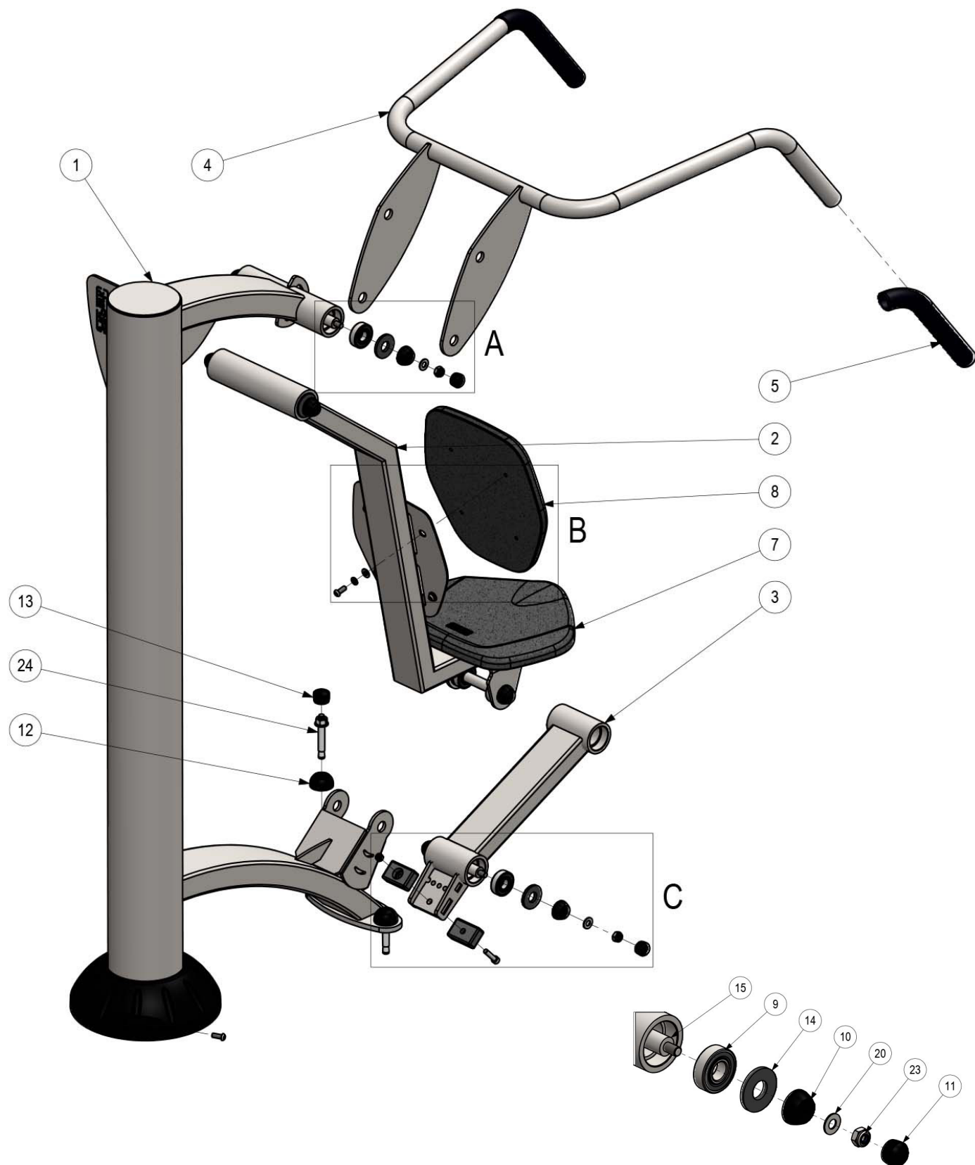
DÉTAIL A
