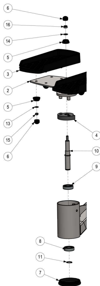
DÉTAIL A
