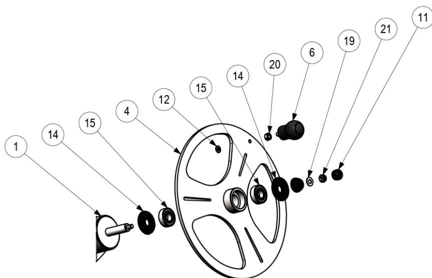
DÉTAIL B
