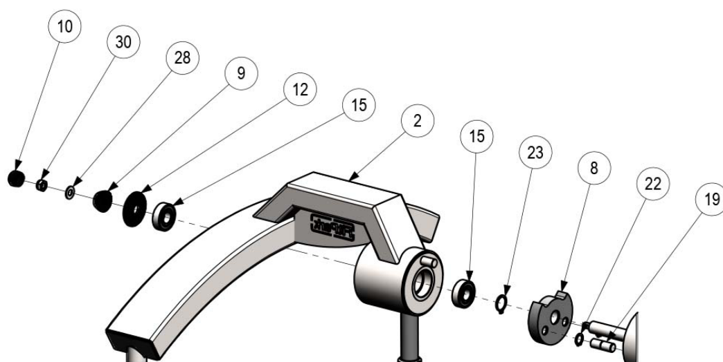
DÉTAIL A
