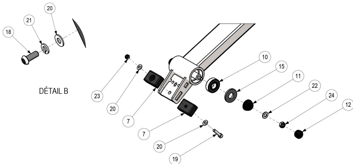
DÉTAIL C
