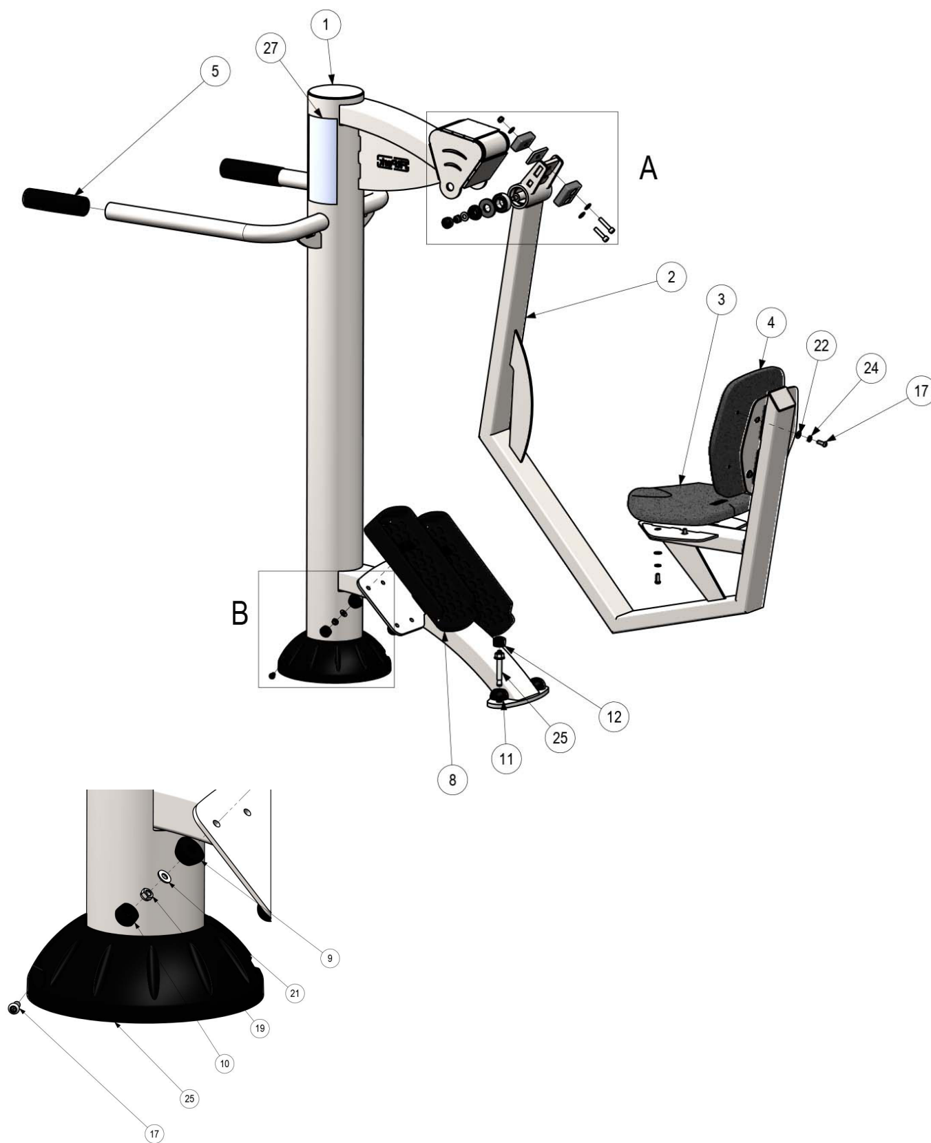
DÉTAIL B
