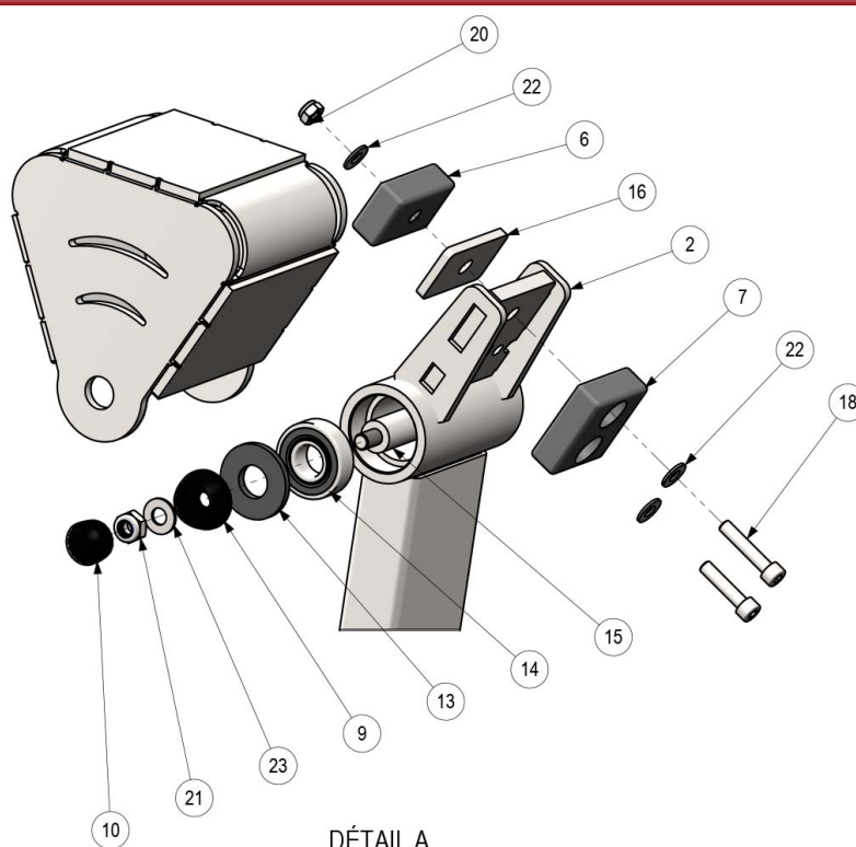
DÉTAIL A
