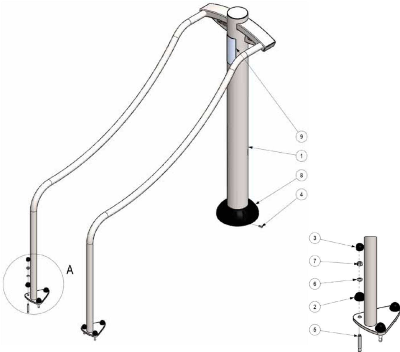
DÉTAIL A
