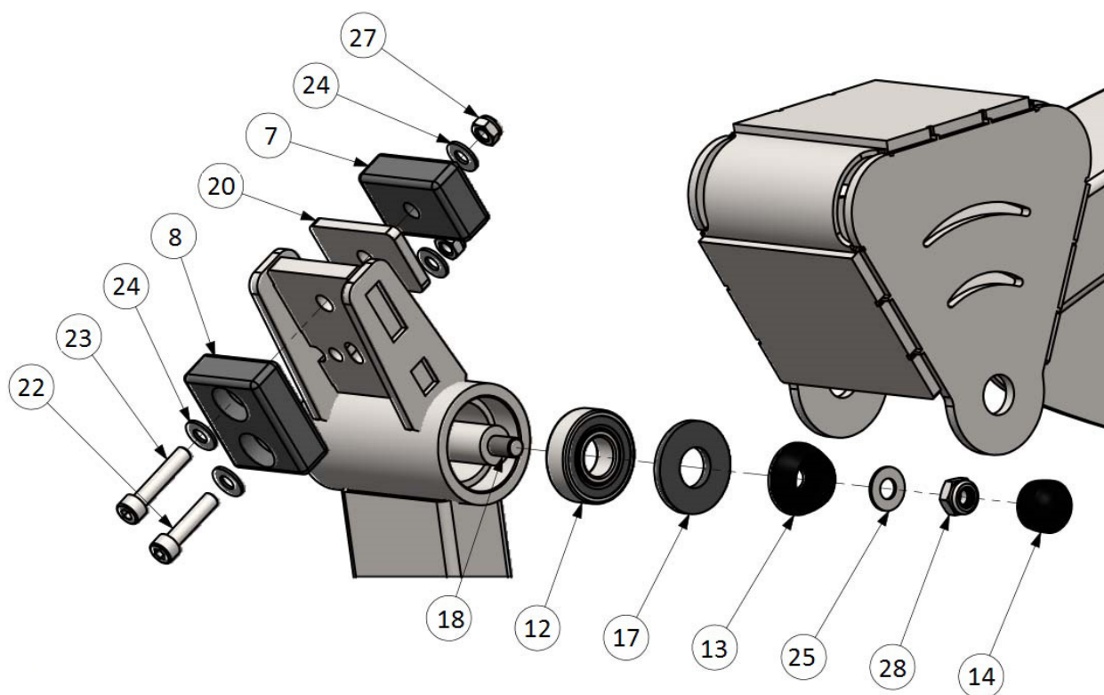
DÉTAIL A
