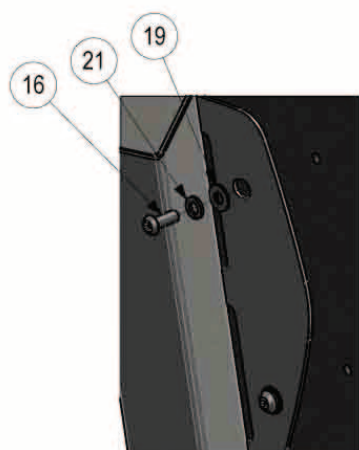
DÉTAIL B
