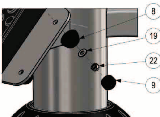
DÉTAIL C
