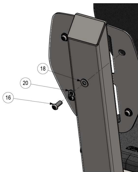
DÉTAIL B
