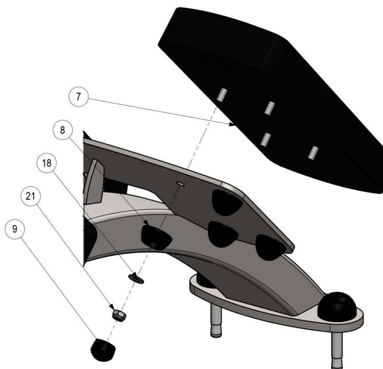
DÉTAIL C
