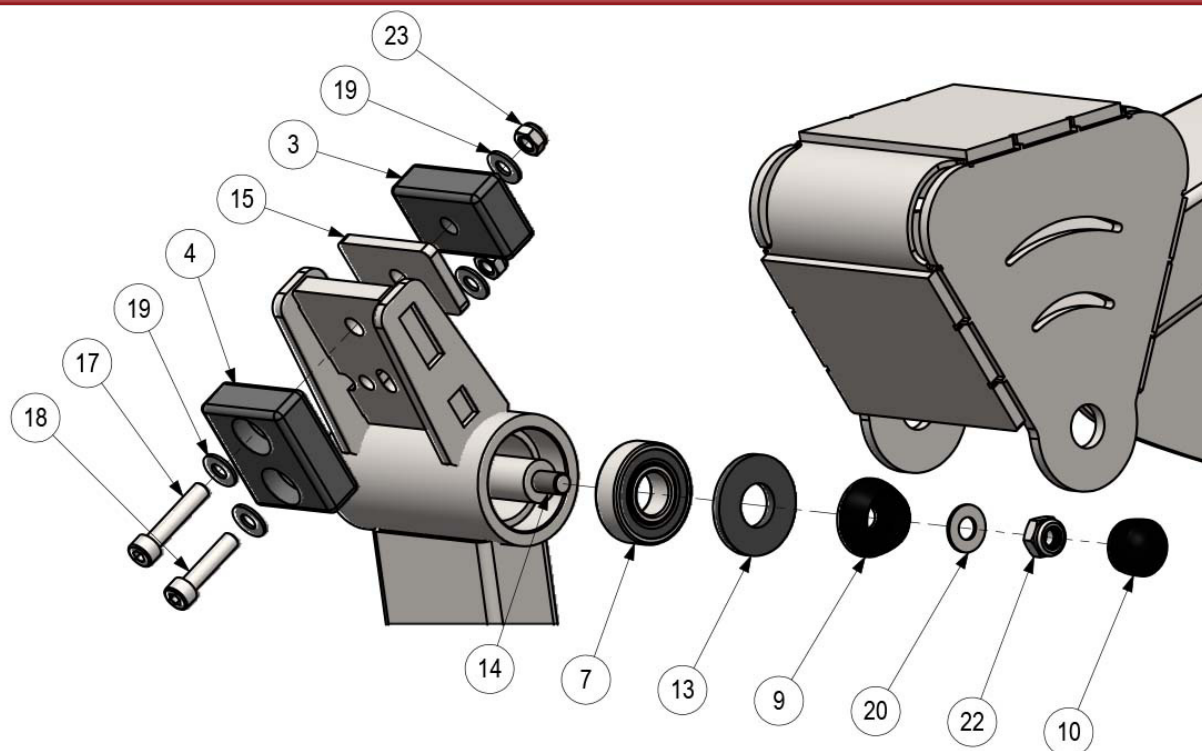
DÉTAIL A
