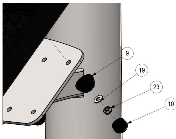
DÉTAIL C
