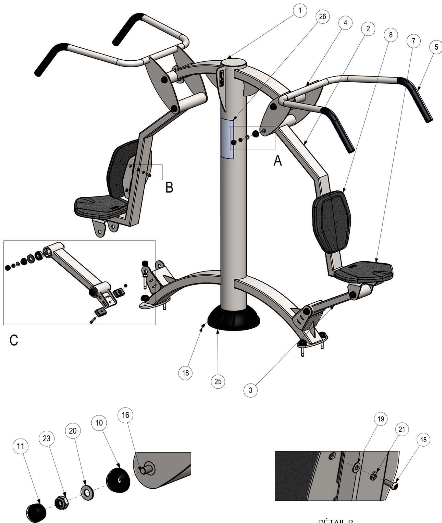
DÉTAIL B
