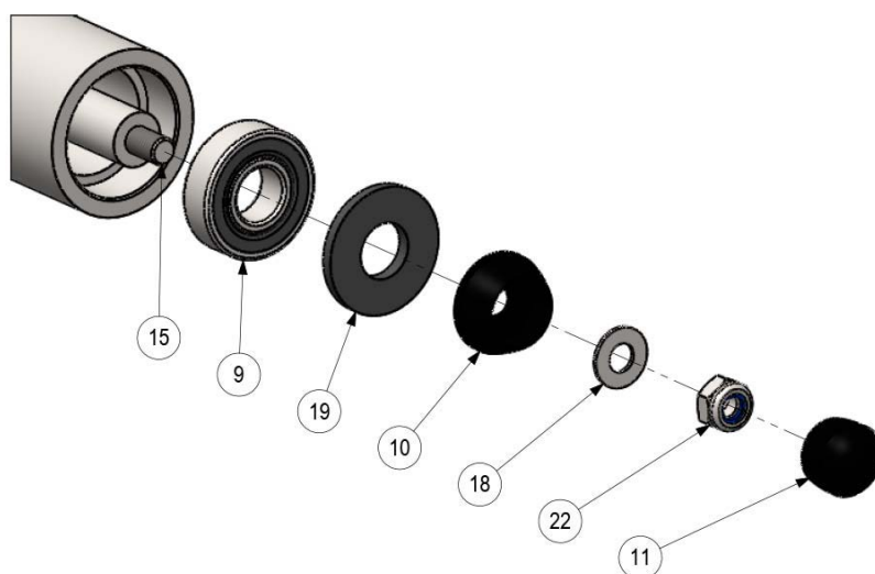
DÉTAIL A
