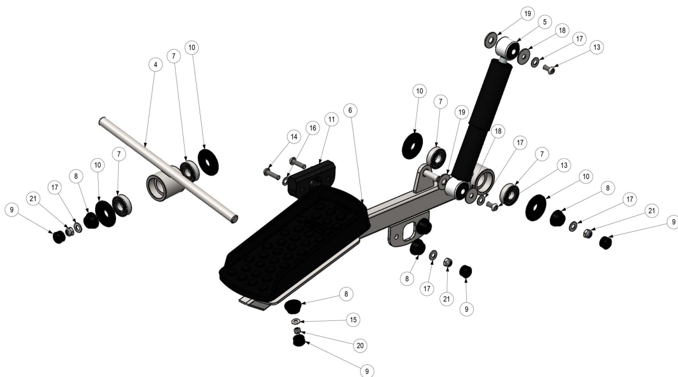
DÉTAIL A
