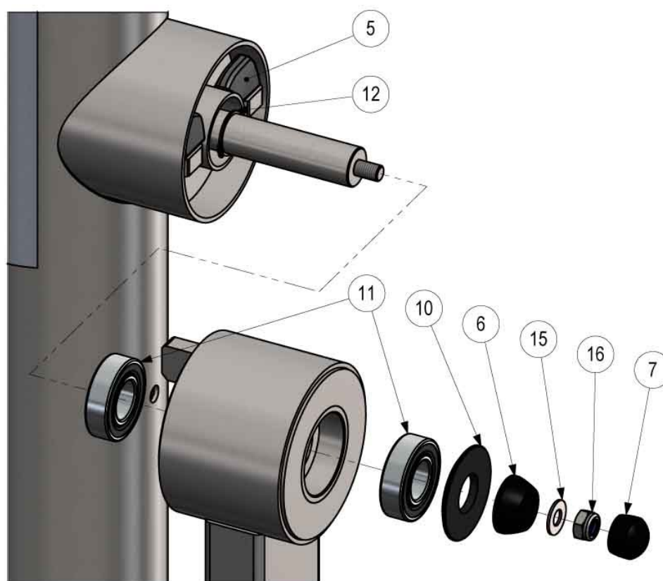
DÉTAIL A
